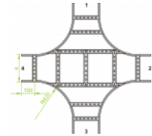
Przy różnych szerokościach drablin należy podać wymiary 1,2,3,4.
